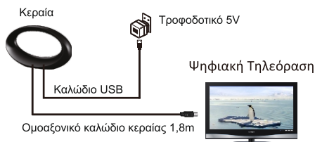
Εικ. 1 Σύνδεση με χρήση του τροφοδοτικού της κεραίας
