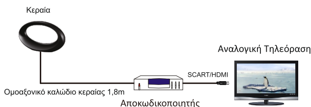
Εικ. 4 Σύνδεση με τροφοδοσία 5V μέσω του Μενού του αποκωδικοποιητή
