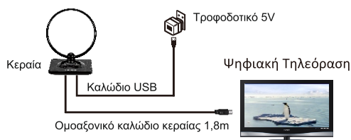
Εικ. 1 Σύνδεση με χρήση του τροφοδοτικού της κεραίας
