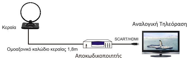
Εικ. 4 Σύνδεση με τροφοδοσία 5V μέσω του Μενού του αποκωδικοποιητή
