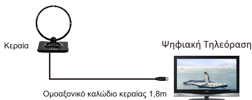
Εικ. 3 Σύνδεση με τροφοδοσία 5V μέσω του Μενού της τηλεόρασης
