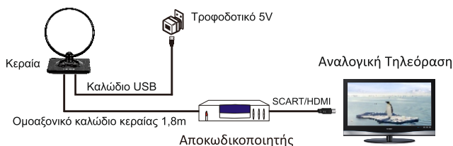
Εικ. 2 Σύνδεση με χρήση του τροφοδοτικού της κεραίας
